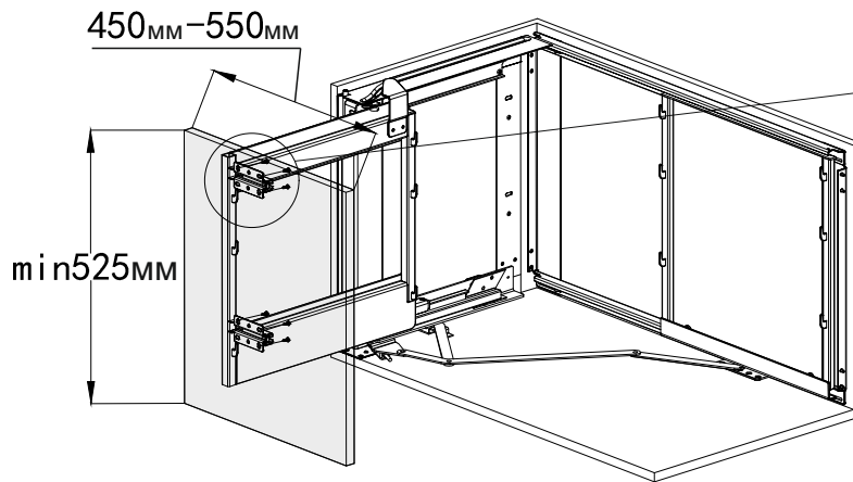
Габаритні розміри фасаду
